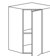
Haut d'angle 60x60 cm 1 porte, 1 étagère Code 005765
