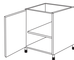
Bas 40/60 cm 1 porte, 1 étagère Code 005771 Code 005773
