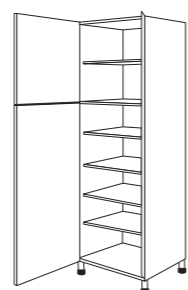
Armoire frigo/rangement 2 portes, 6 étagères, Caisson 475048 Coloris façades 489748+489702
