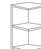
Étagère haute H. 70,7 - P. 33,5 cm 401180
