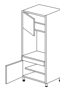
Four encastrable - 2 portes, 2 étagères, 1 tiroir, 1 bandeau de calfeutrement Caisson 475048 Coloris façades 489711+489743+489745
