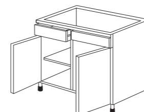
Bas 80 cm - 2 portes, 1 étagère, 2 tiroirs Caisson 475014 Coloris façades 489709x2
