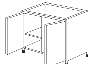
Bas 120 cm - 2 portes, 1 étagère, Caisson 475015 Coloris façades 489702x2
