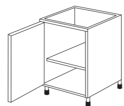
Bas 40 cm - 1 porte, 1 étagère Caisson 475009 Coloris façades 489701
