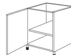
Bas 60 cm sous-évier ou plaque 1 porte, 1 étagère - Caisson 475011 Coloris façades 489702
